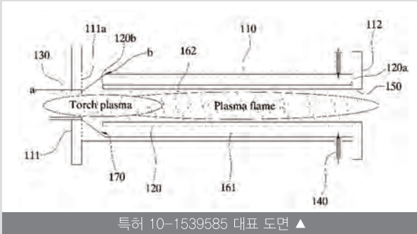
폐가스를 플라즈마 화염 출구로 유입하여 처리 효율을 높이는 기술의 개념도 ▲
