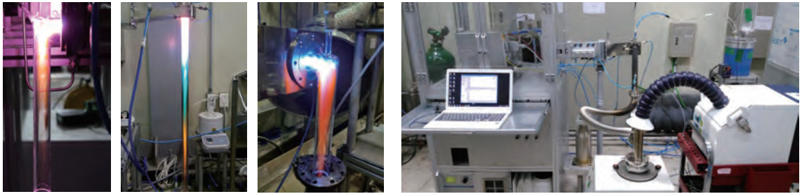
스웰 형태의 플라즈마 내부로 개질 대상 물질을 쉽게 주입할 수 있는 플라즈마 반응기 시제품 ▲
