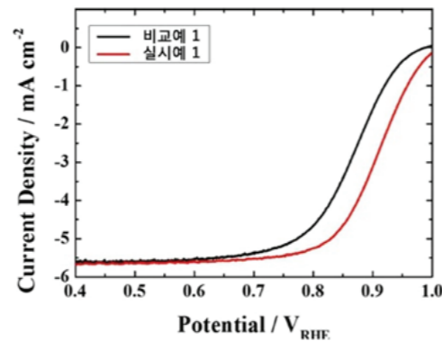
제조된 Pt/C(질소 원자 도핑) 촉매 및 비교예에 따라 제조된 Pt/C 촉매의 반쪽 전지(Half-cell)를 통해 산소환원반응(ORR) 분극 초기 성능 비교 그래프
